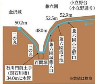
「伏越之理」のイメージ 「伏越之理」—倒虹虹連通管。
